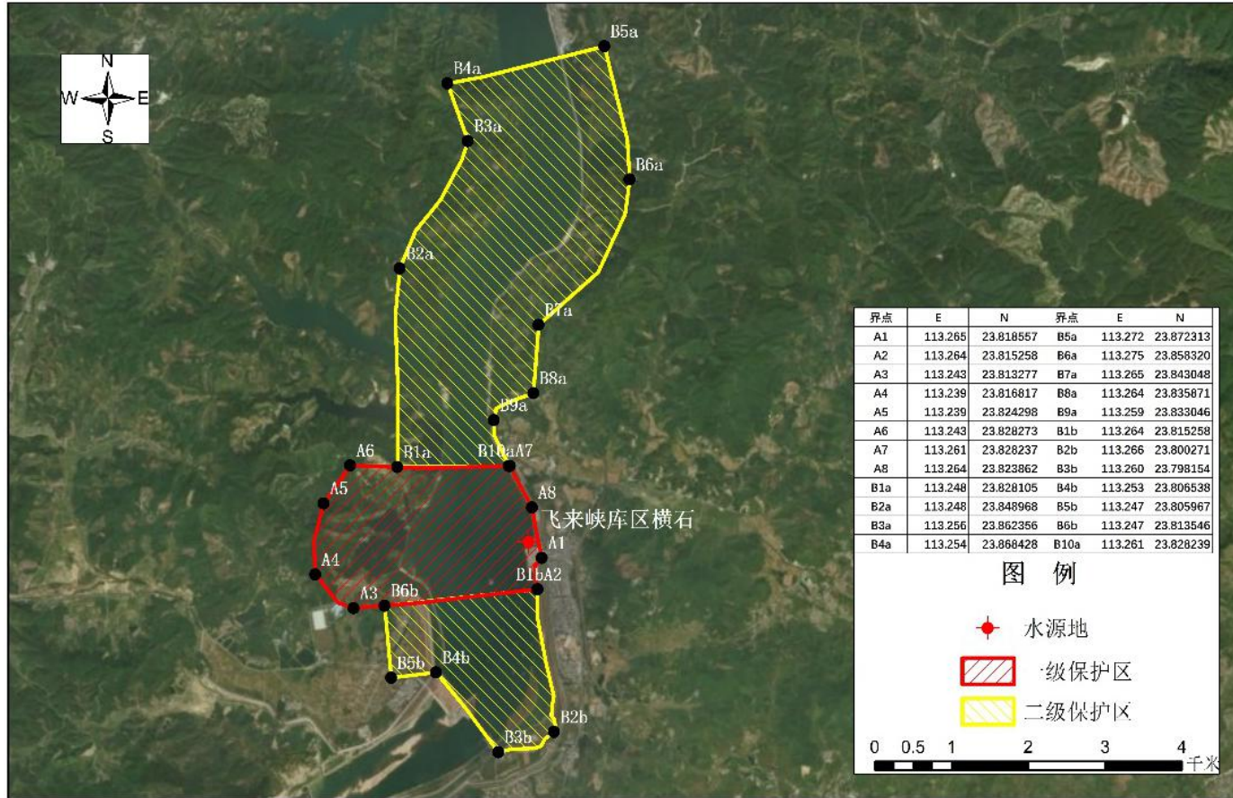
清城区飞来峡镇飞来峡横石水源保护区划分定界图
